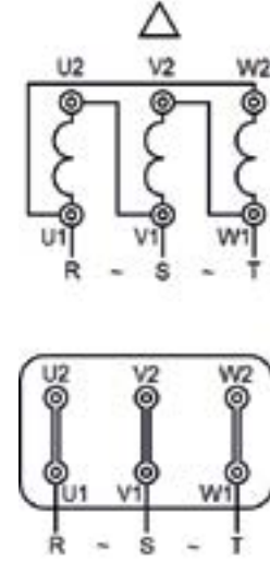
MOTORES TRIFÁSICOS 400/690
